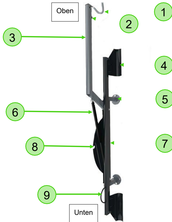
Abbildung 2 Ausführungsvariante Bicyclejack
